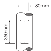
SERVICE DOOR
